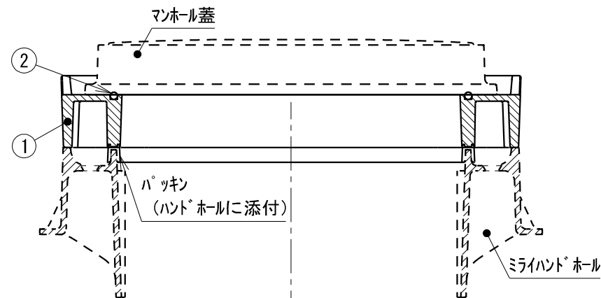
施工状態参考図
