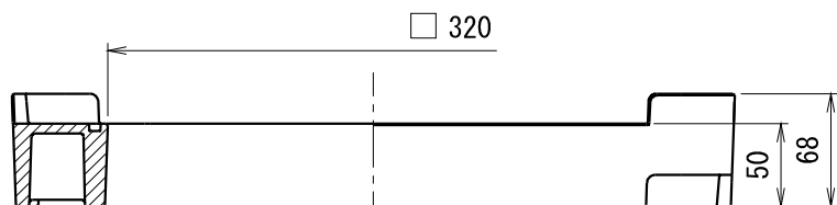
断面 A-A
